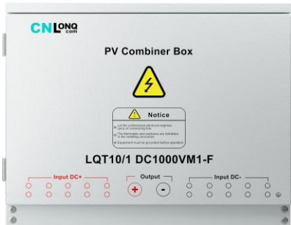
510*650*180mm
