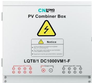
510*510*180mm
