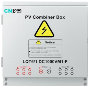
450*450*180mm
