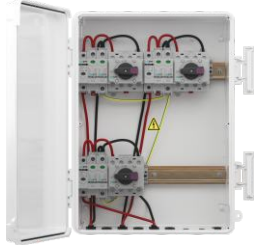
LQX-N3/3DC1000VQ
