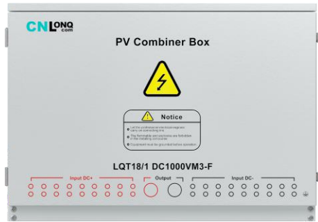
610*850*220mm
