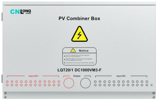
610*950*220mm
