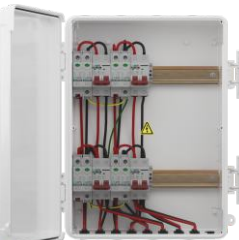
LQX-N4/4DC500VBS
