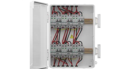
LQX-N6/6DC600VLS
