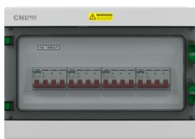
LQX-4/4DC1000VBB
