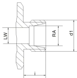
DIN 2353 LR
