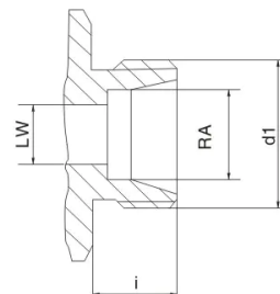
DIN 2353 SR
