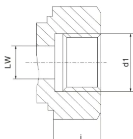
ISO 228
