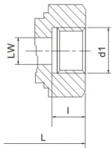
公制内螺纹
