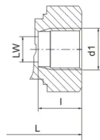
ISO7-1 内螺纹
