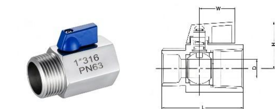
迷你球阀 MINI Ball Valve
